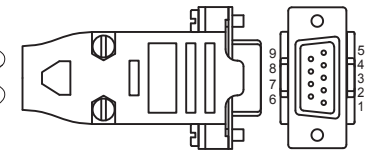
DB-9 Connector (RS-232)
